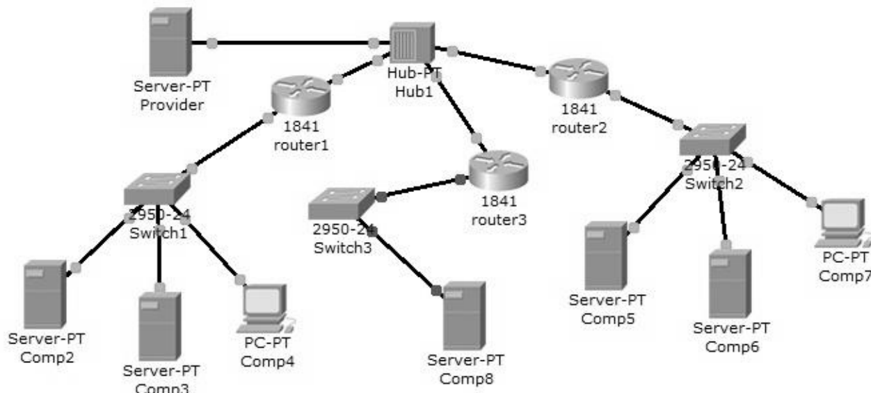
Рис. 18 Схема сети.
