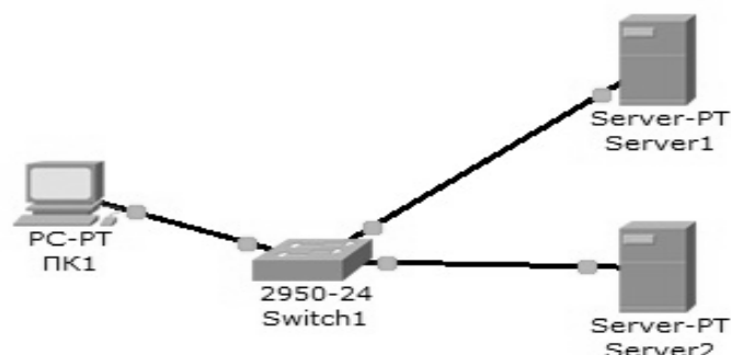
Рис. 10 Схема сети.
