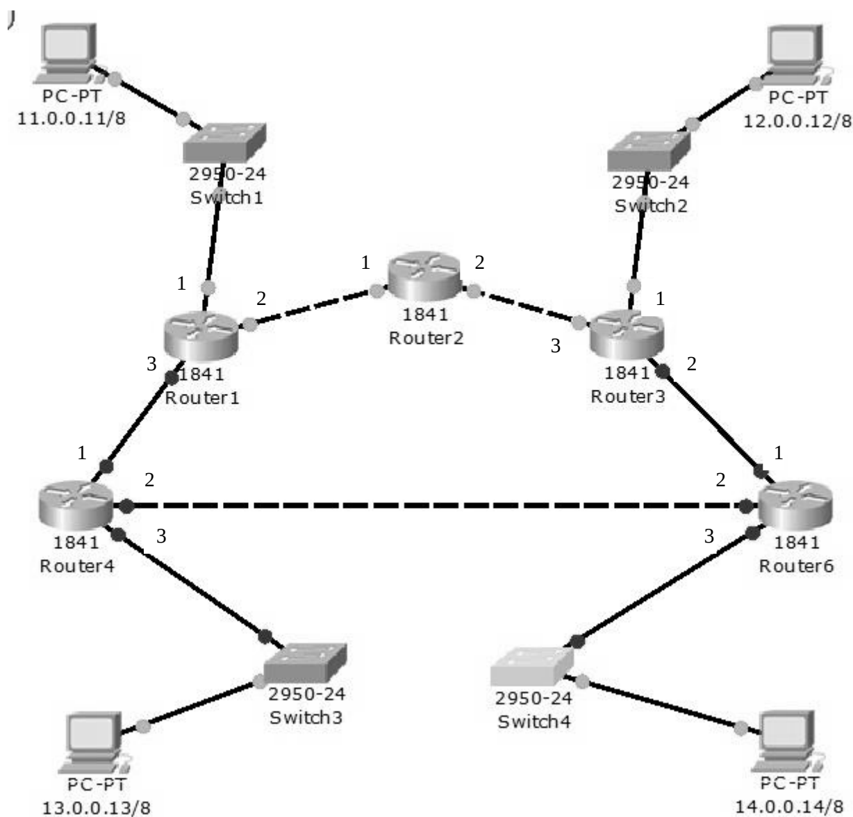
Рис. 22 Схема сети.
