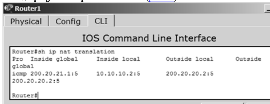
Рис. 36 Адреса: глобальный, внутренний, внешний
