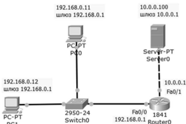
Рис. 24 Схема сети.
