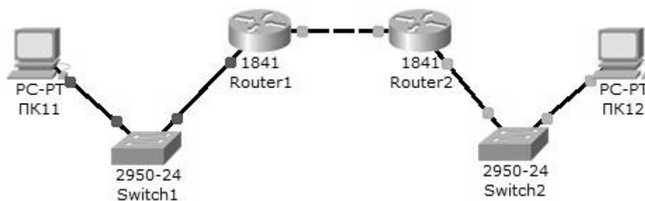
Рис. 21 Схема сети.
