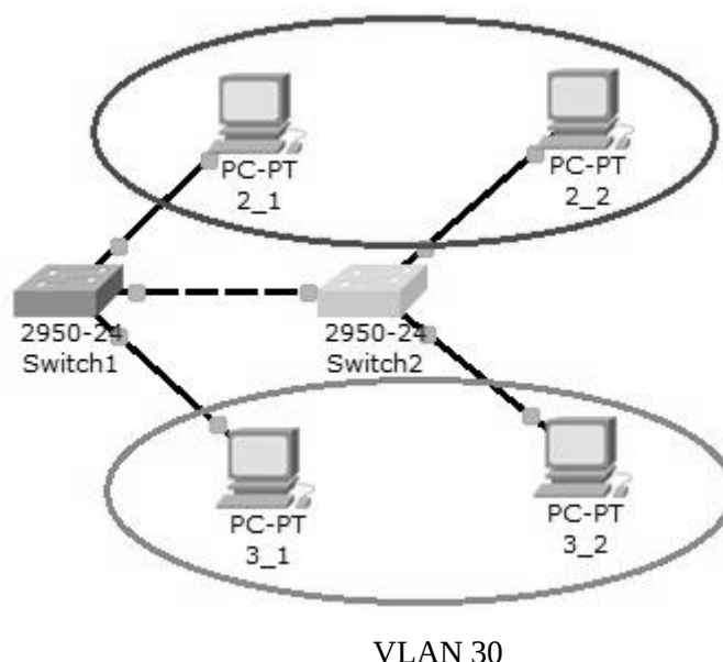
Рис. 43 Схема сети.
