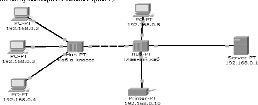
Рис. 1 Схема сети.
