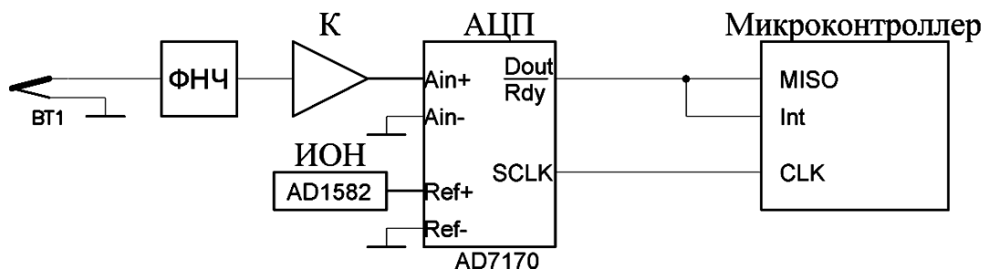
Рис.1. Функциональная схема информационного канала.
